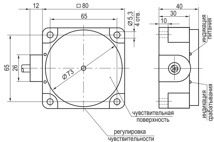
Габаритный чертеж
