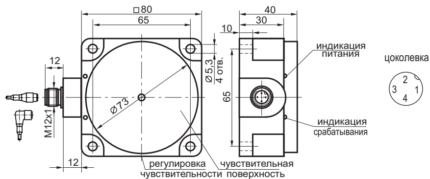
Габаритный чертеж
