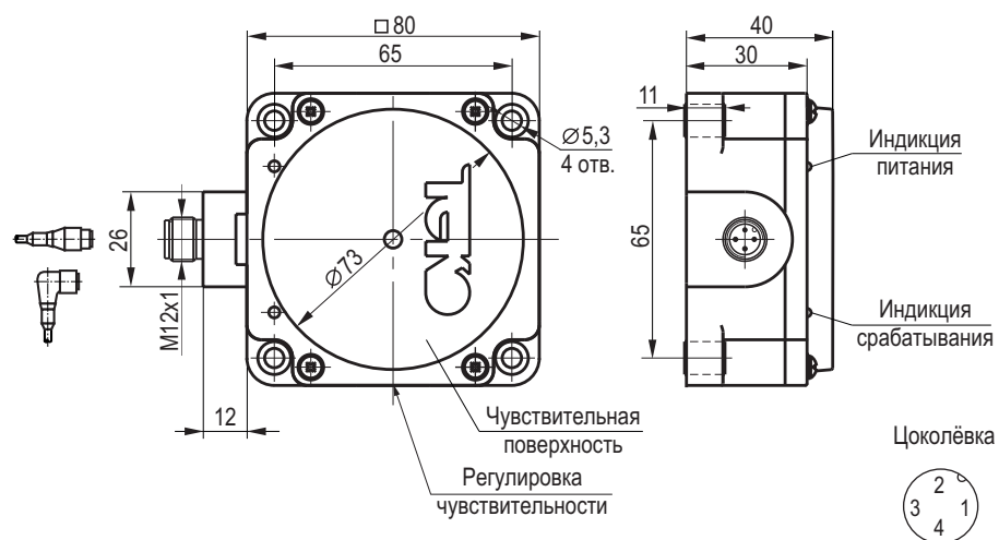
Габаритный чертеж
