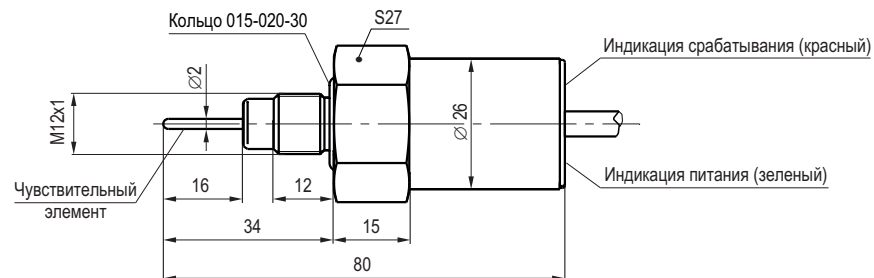
Габаритный чертеж.
