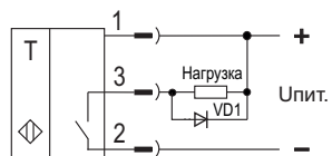
Схема подключения
