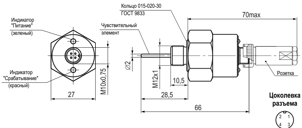
Габаритный чертеж
