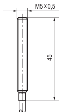
Габаритный чертеж
