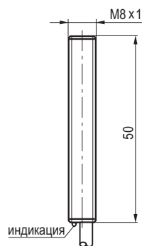
Габаритный чертеж
