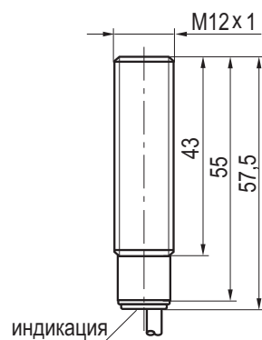
Габаритный чертеж
