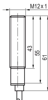
Габаритный чертеж
