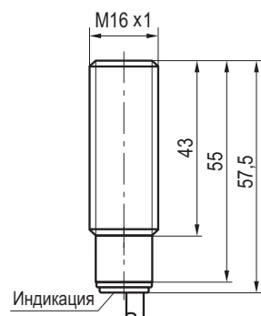
Габаритный чертеж
