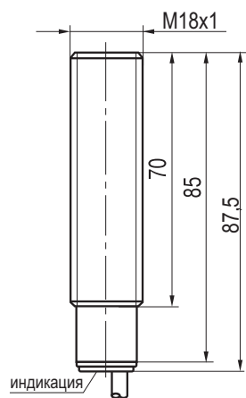
Габаритный чертеж
