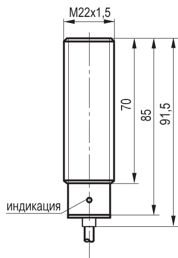
Габаритный чертеж
