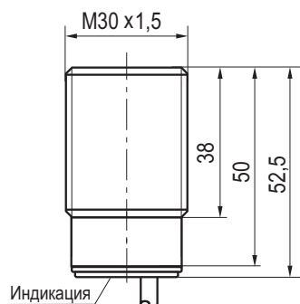
Габаритный чертеж
