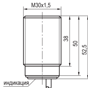
Габаритный чертеж
