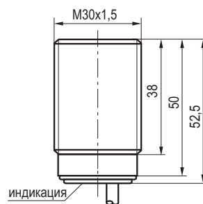
Габаритный чертеж
