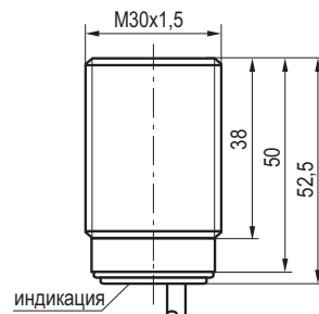
Габаритный чертеж
