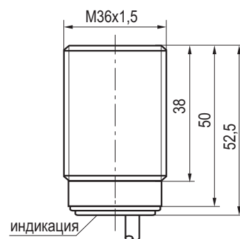
Габаритный чертеж
