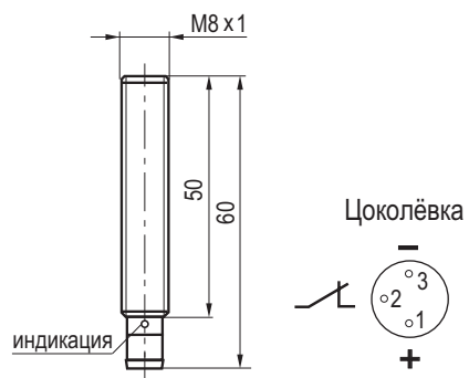
Габаритный чертёж
