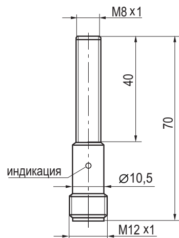
Габаритный чертеж
