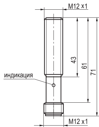
Габаритный чертеж
