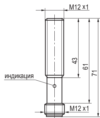
Габаритный чертеж
