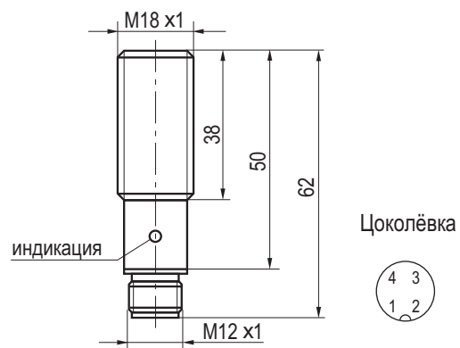
Габаритный чертеж
