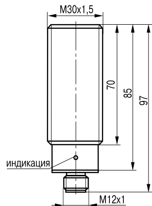
Габаритный чертеж
