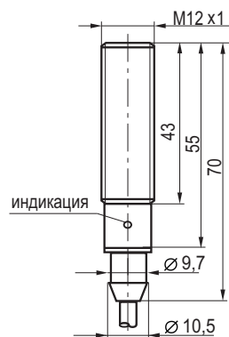
Габаритный чертеж
