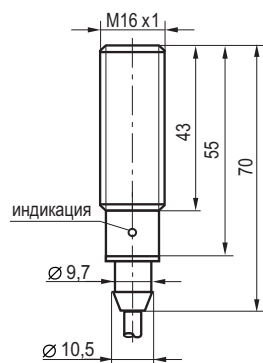
Габаритный чертеж
