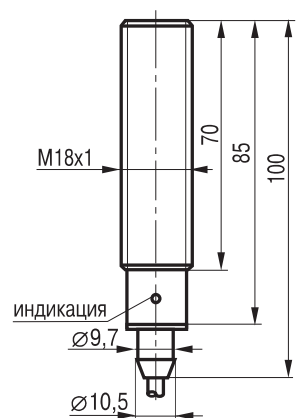
Габаритный чертеж
