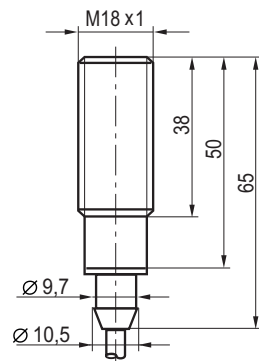
Габаритный чертеж
