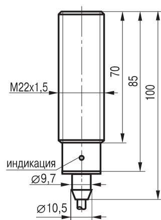
Габаритный чертеж
