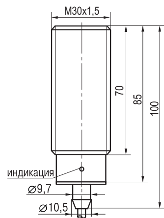
Габаритный чертеж
