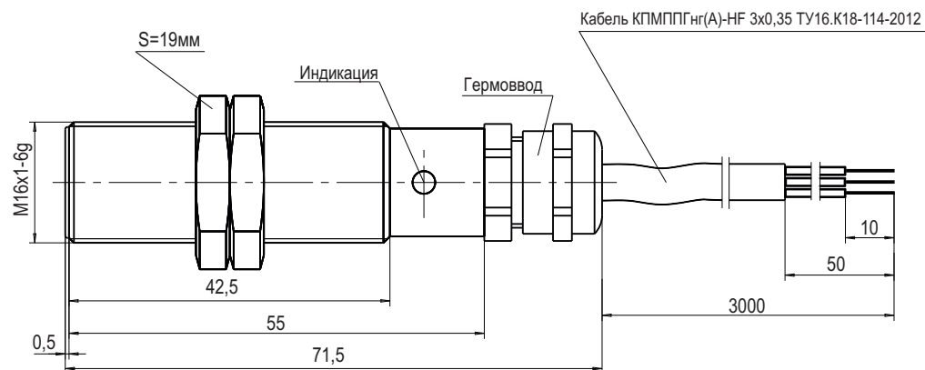
Габаритный чертеж
