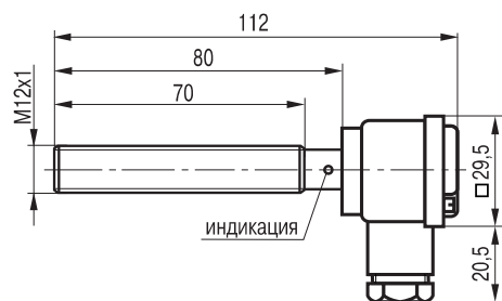
Габаритный чертеж
