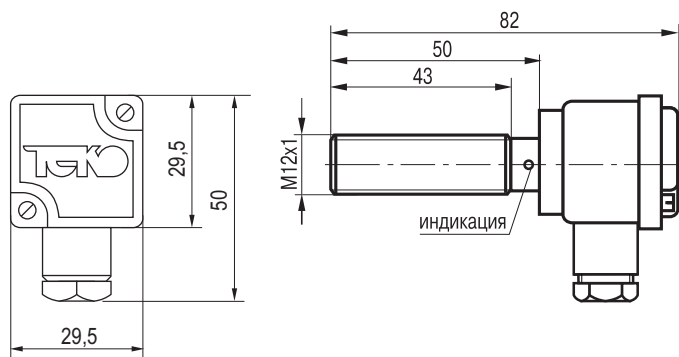
Габаритный чертеж
