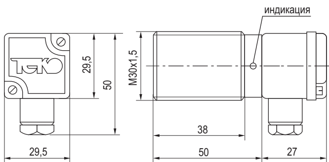
Габаритный чертёж
