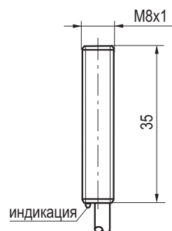
Габаритный чертеж
