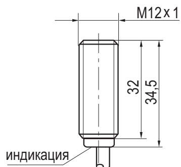
Габаритный чертеж
