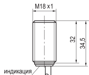
Габаритный чертеж
