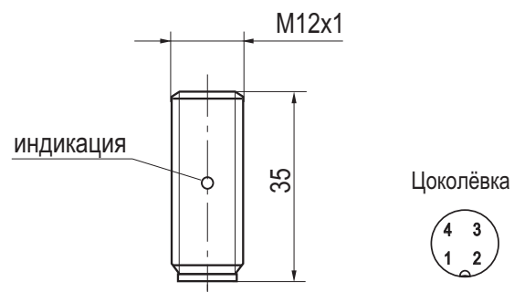
Габаритный чертеж
