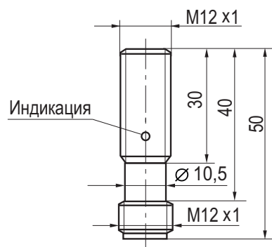
Габаритный чертеж
