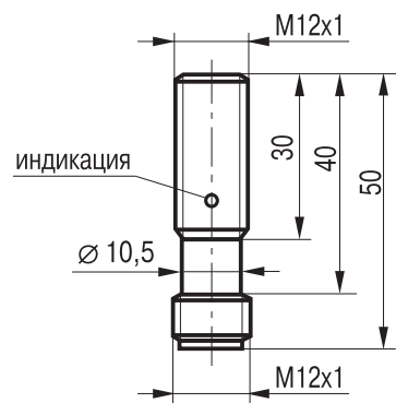
Габаритный чертеж
