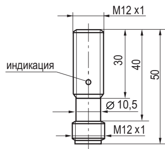
Габаритный чертёж
