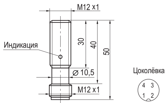
Габаритный чертеж
