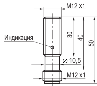
Габаритный чертеж
