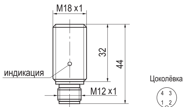
Габаритный чертеж
