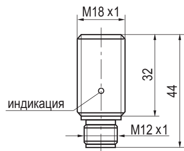
Габаритный чертеж
