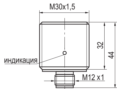
Габаритный чертеж
