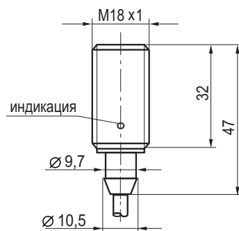
Габаритный чертеж
