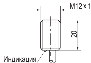
Габаритный чертеж
