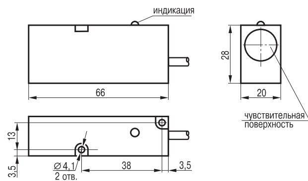
Габаритный чертеж
