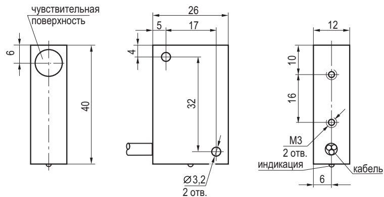
Габаритный чертёж
