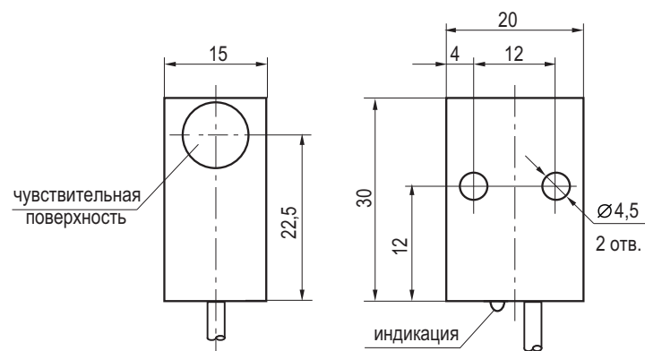
Габаритный чертёж
